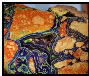
Azurite Brecchia
